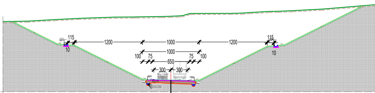
НОРМАЛНИ ПРОФИЛ У УСЕКУ
