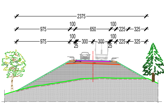
НОРМАЛНИ ПРОФИЛ У НАСИПУ
