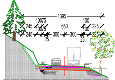
НОРМАЛНИ ПРОФИЛ У ЗАСЕКУ
