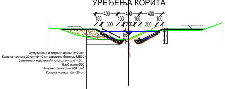
НОРМАЛНИ ПОПРЕЧНИ ПРОФИЛ УРЕЂЕЊА КОРИТА
