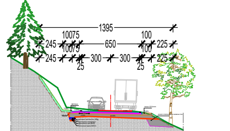
НОРМАЛНИ ПРОФИЛ У ЗАСЕКУ
