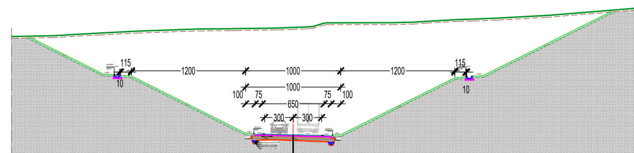
НОРМАЛНИ ПРОФИЛ У УСЕКУ
