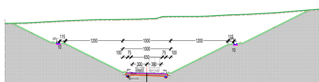
НОРМАЛНИ ПРОФИЛ У УСЕКУ
