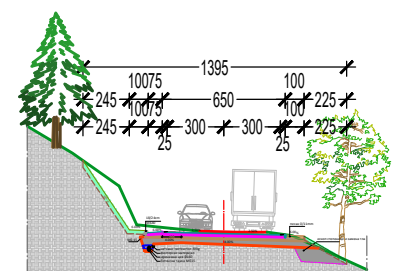
НОРМАЛНИ ПРОФИЛ У ЗАСЕКУ
