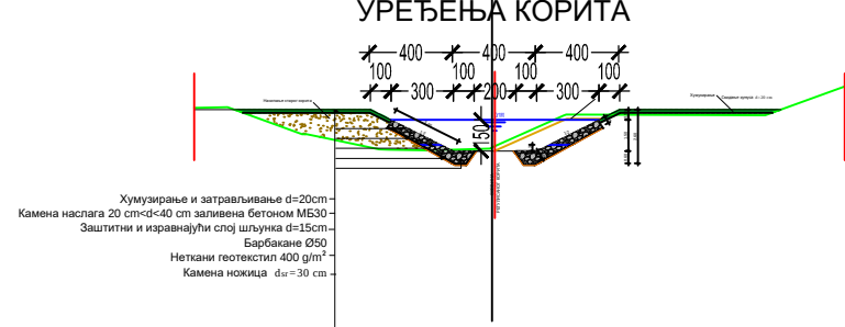
НОРМАЛНИ ПОПРЕЧНИ ПРОФИЛ УРЕЂЕЊА КОРИТА
