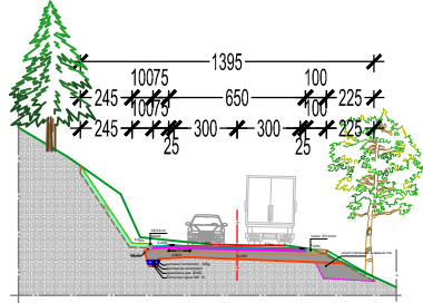
НОРМАЛНИ ПРОФИЛ У ЗАСЕКУ
